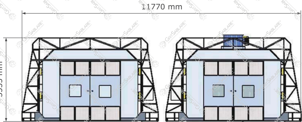
CAMERA DE SABLARE
