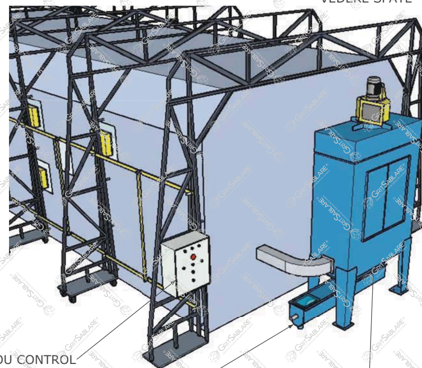
VEDERE SPATE
